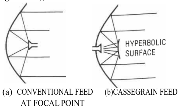
Figure 38. Parabolic antennas.
